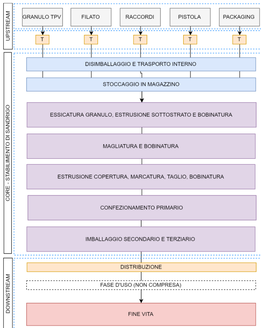
Figura 1 Schema del processo produttivo relativo ai prodotti della famiglia FITT Force
